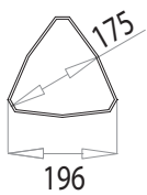
SEZIONE | SECTION B.B
