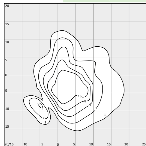
LA4-9 (LA4-9.Idt) Fußgängerüberweg LPH: 6m 4500 lm Von seitlicher Mastposition rechts
