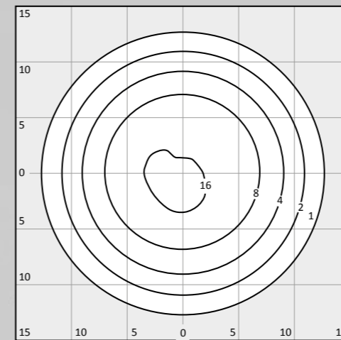
LA4-C (LA4-C.Idt) LPH: 6m 4500 lm
