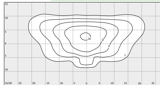
LA4-2 (LA4-2.Idt) Verkehrsstraße (ME-Klasse) LPH: 6m 4500 lm Von seitlicher Mastposition
