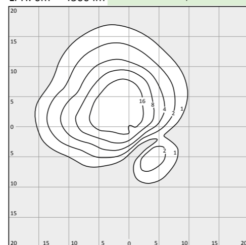
LA4-B (LA4-B.Idt) Fußgängerüberweg LPH: 6m 4500 lm Von seitlicher Mastposition links
