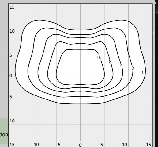
LA4-8 (LA4-8.Idt) LPH: 6m 4500 lm
