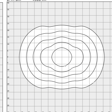
MR doppelasymmetrisch C0-C180 (150.300.ltd) LPH: 6m 4500 lm
