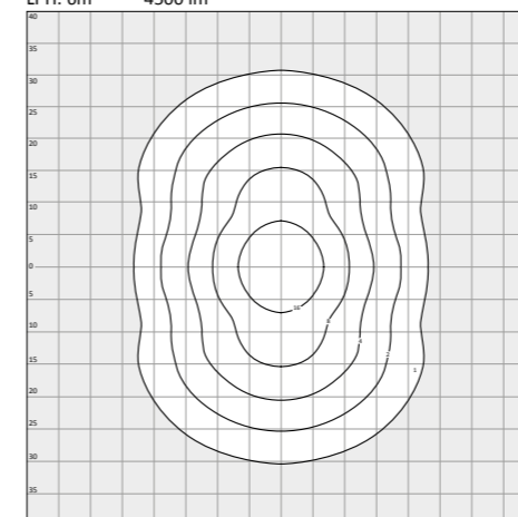
MR doppelasymmetrisch C90-C270 (150.200.ltd) LPH: 6m 4500 lm
