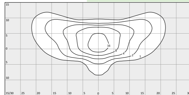
LA4-2 (LA4-2.Idt) Verkehrsstraße (ME-Klasse) LPH: 6m 4500 lm Von seitlicher Mastposition
