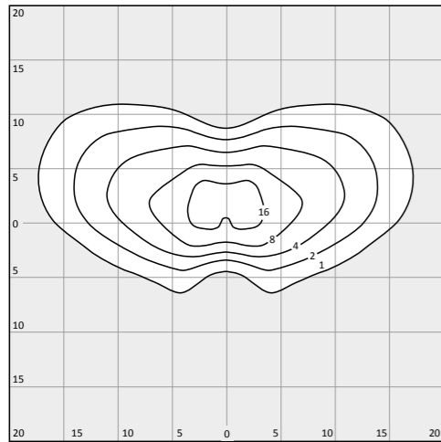
Straße mit rückwärtigem Bereich Von seitlicher Mastposition
