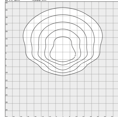
MR asymmetrisch C90 (150.100.ltd) LPH: 6m 4500 lm
