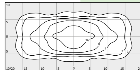
LA4-4 (LA4-4.Idt) Verkehrsstraße LPH: 6m 4500 lm Überspannleuchte mittig
